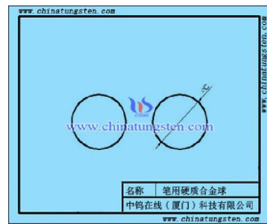
筆用硬質合金球圖紙
