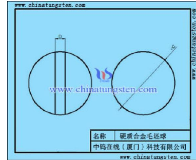
硬質合金毛坯球圖紙
